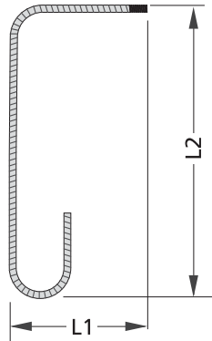
Typ/Type Z G
