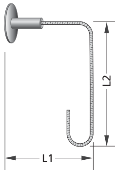
Typ/Type Z C
